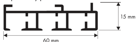
trojdrážkový profil
