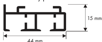
dvoudrážkový profil
