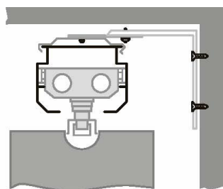
b) na stěnu (pomocí konzole a klipu)
